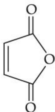
Maleic anhydride
