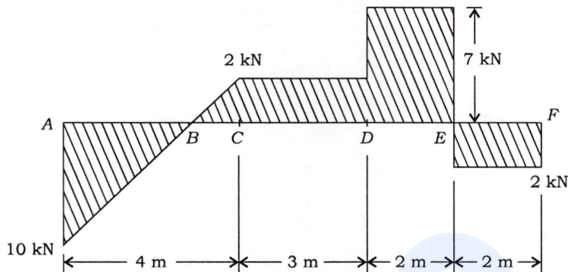
अपरूपण बल आरेख
